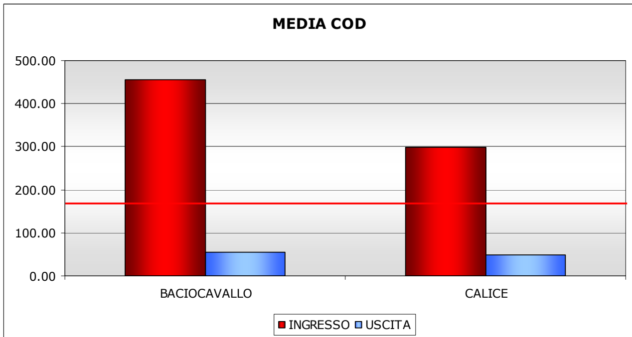
Fig.I. 78 – Confronto tra le concentrazioni medie di COD in entrata ed in uscita agli impianti di depurazione – Elaborazione dati GIDA
