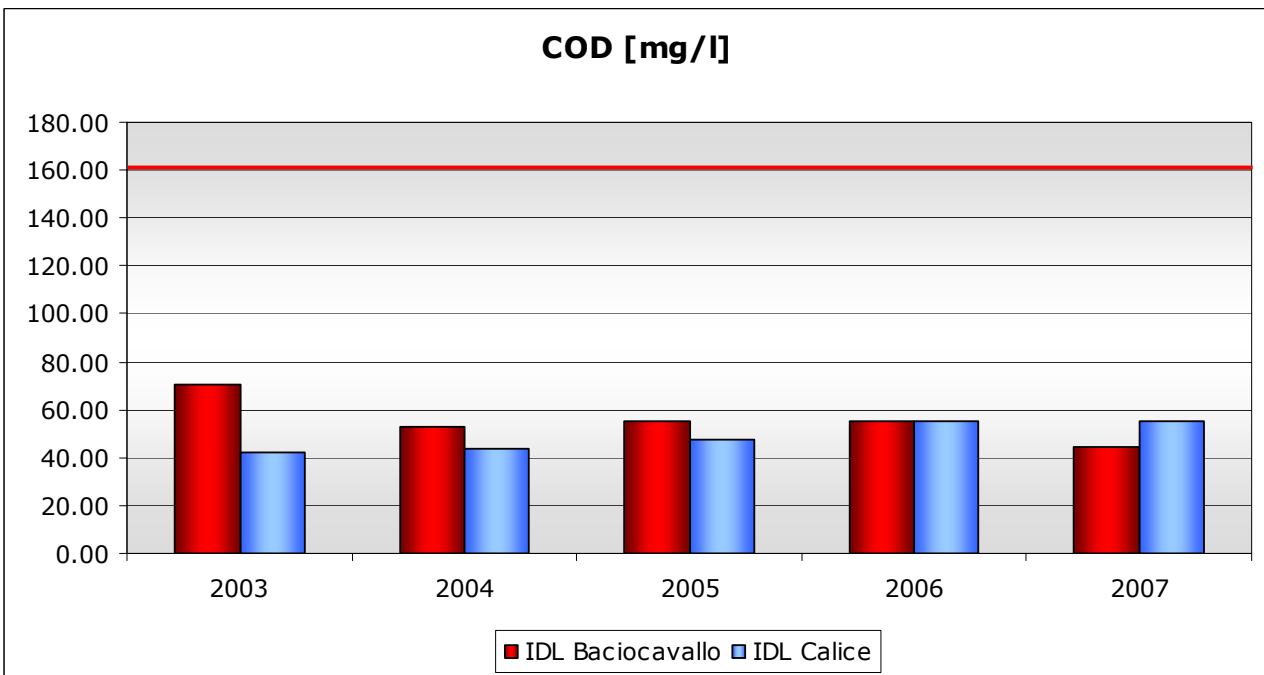
Fig.I. 76– Monitoraggio delle concentrazioni di COD negli scarichi degli impianti di depurazione – Elaborazione dati GIDA
