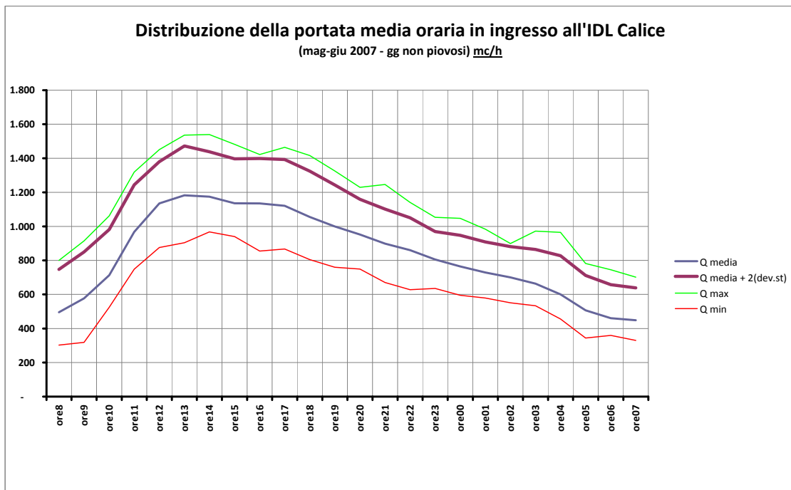
Fig.I. 73 - Distribuzione portata oraria in ingresso IDL Calice (Publiacqua Ing)
