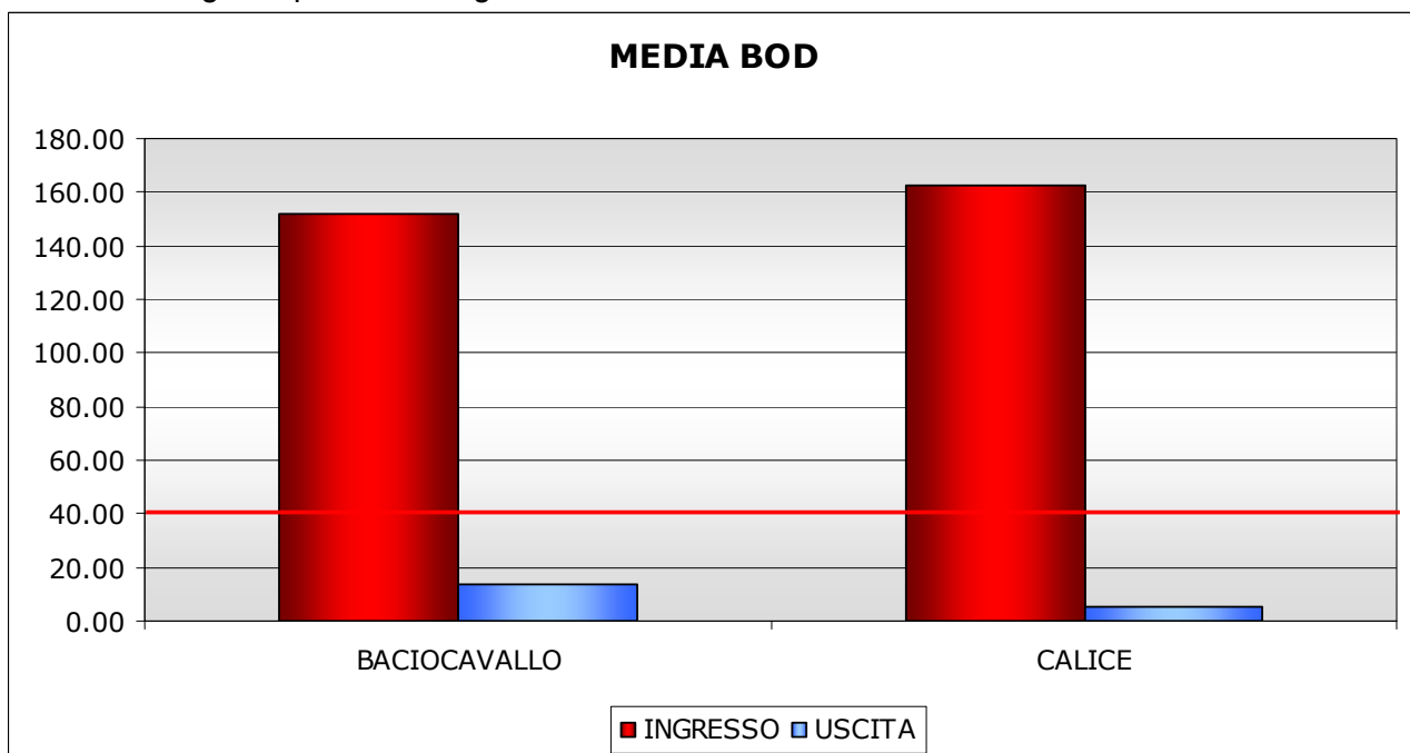
Fig.I. 79 - Confronto tra le concentrazioni medie di BOD in entrata ed in uscita agli impianti di depurazione – Elaborazione dati GIDA
