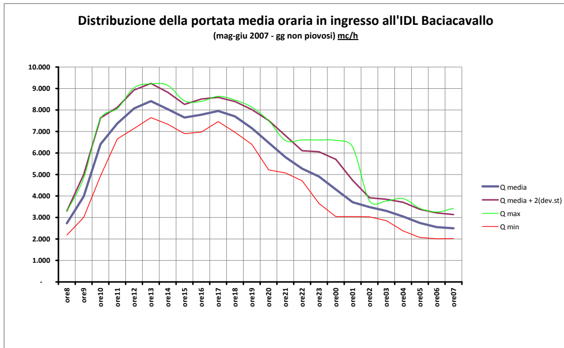
Fig.I. 71 - Distribuzione portata oraria in ingresso IDL Baciacavallo (Publiacqua Ing)
