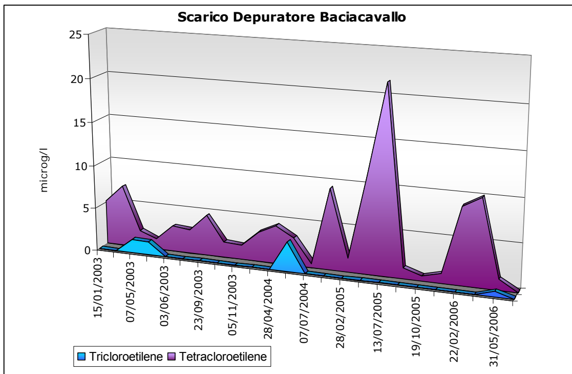
Fig.I. 92 Andamento concentrazioni tricloroetilene e tetracloroetilene nelle acque di scarico del depuratore Baciacavallo (ARPAT)
