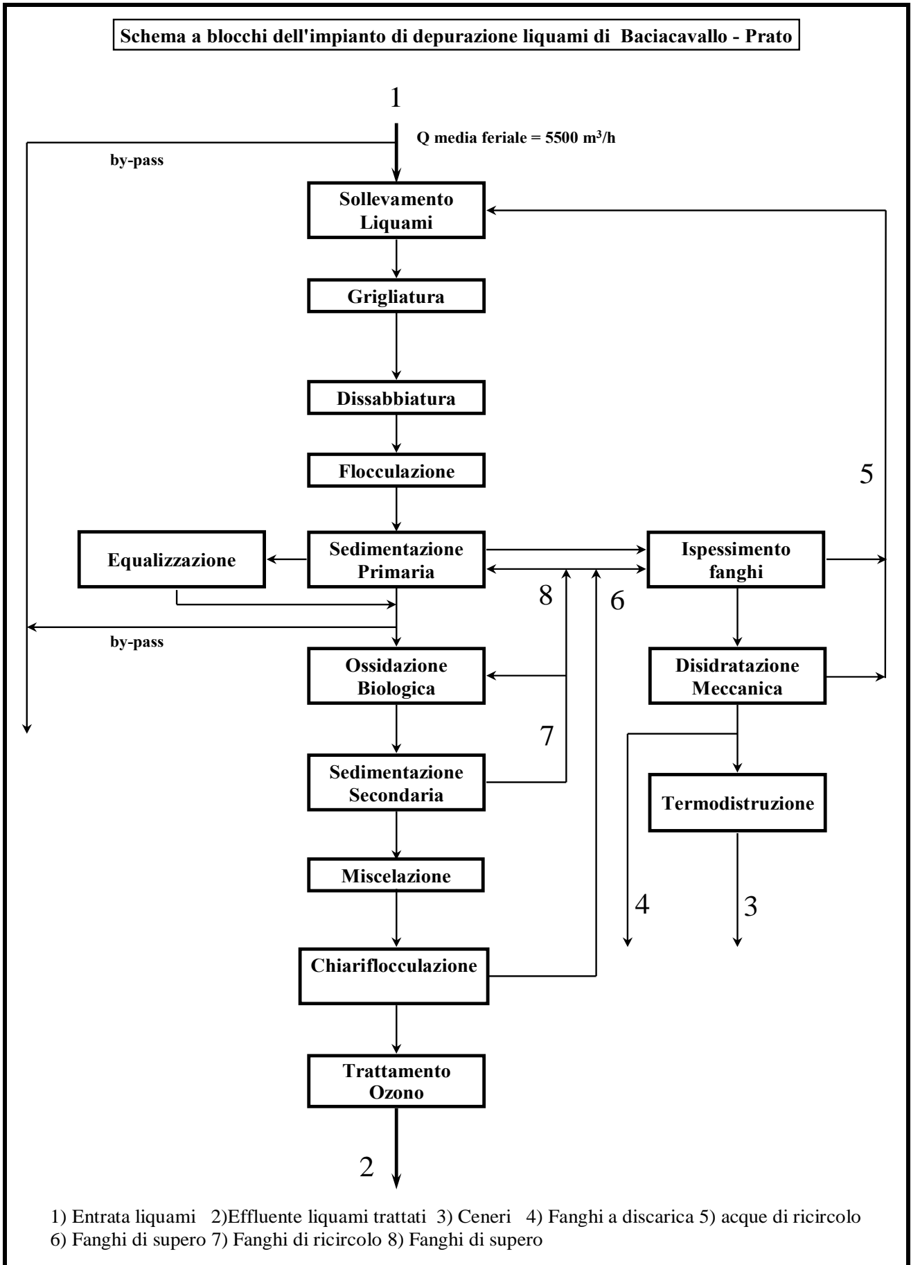
Fig.I. 72 – Impianto di depurazioni liquami Baciacavallo
