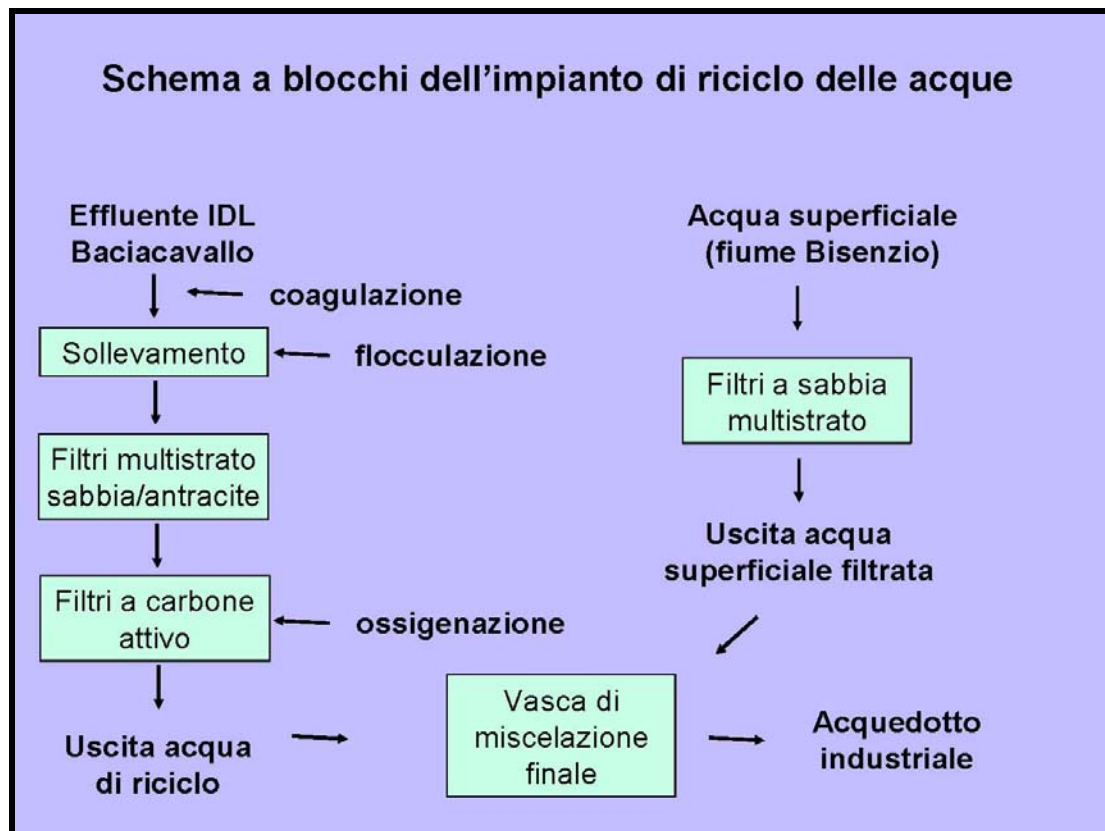
Fig.I. 65 – Impianto riciclo acque (GIDA)
